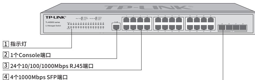
图1-8 TL-NS650-24G4F前面板示意图
