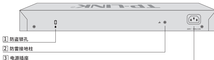
图1-18 后面板示意图
