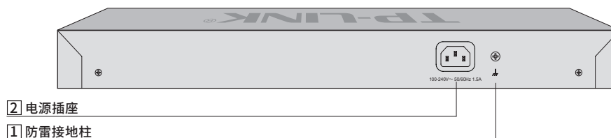
图1-17 后面板示意图
