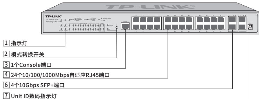
图1-10 TL-NS660-24GP4T前面板示意图
