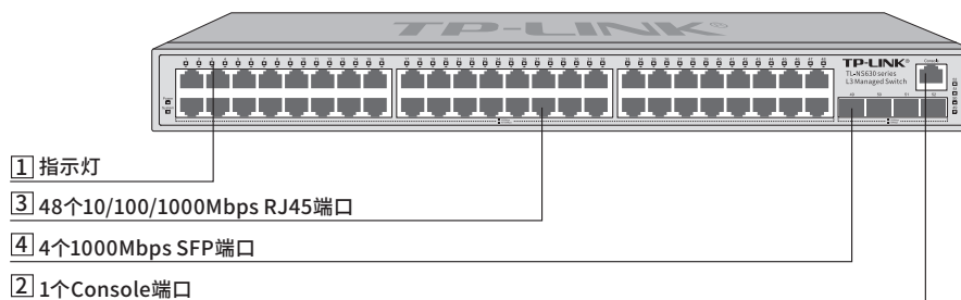
图1-9 TL-NS630-48G4F前面板示意图
