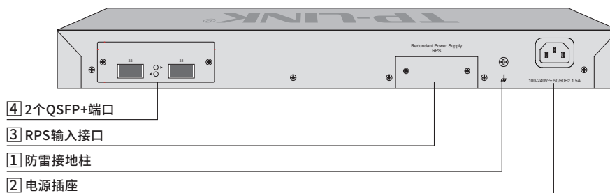
图1-15 TL-NS680-24F4G4T2Q后面板示意图
