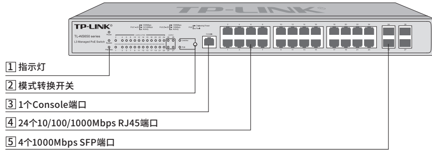
图1-12 TL-NS650-24GP4F前面板示意图
