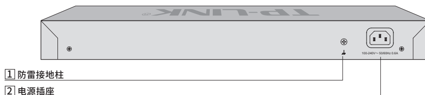
图1-16 后面板示意图
