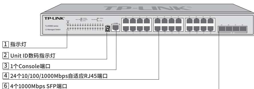
图1-6 TL-NS660-24G4F前面板示意图
