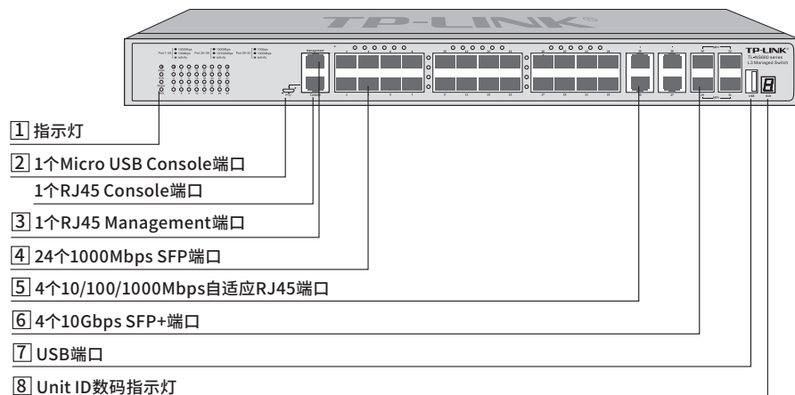
图1-3 TL-NS680-24F4G4T2Q前面板示意图
