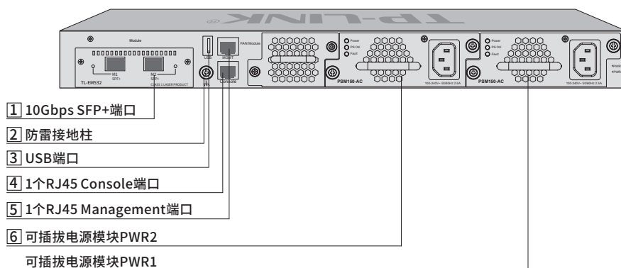
图1-14 TL-NS680-48G4F4T后面板示意图
