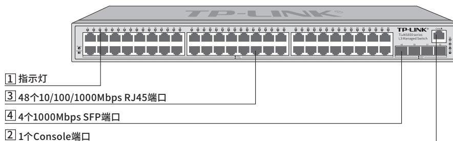
图1-7 TL-NS650-48G4F前面板示意图
