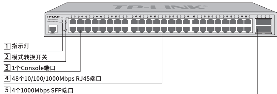
图1-11 TL-NS650-48GP4F前面板示意图
