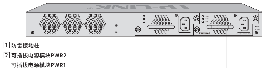
图1-13 TL-NS680-24T2Q后面板示意图
